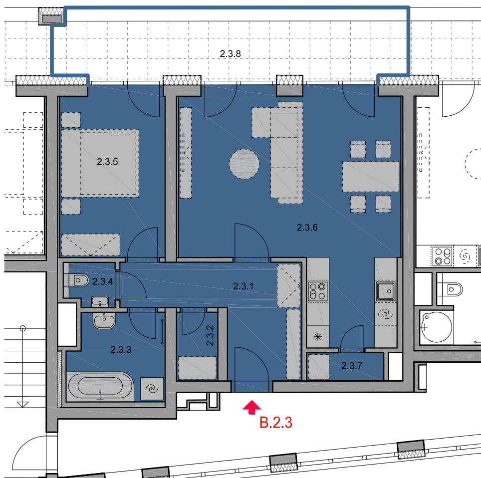
PŮDORYS 1:100
