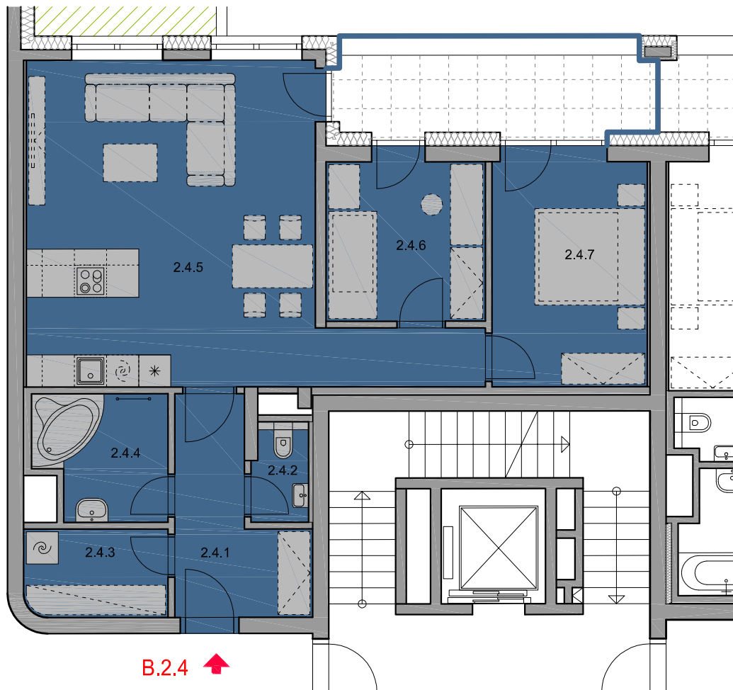
PŮDORYS 1:100
