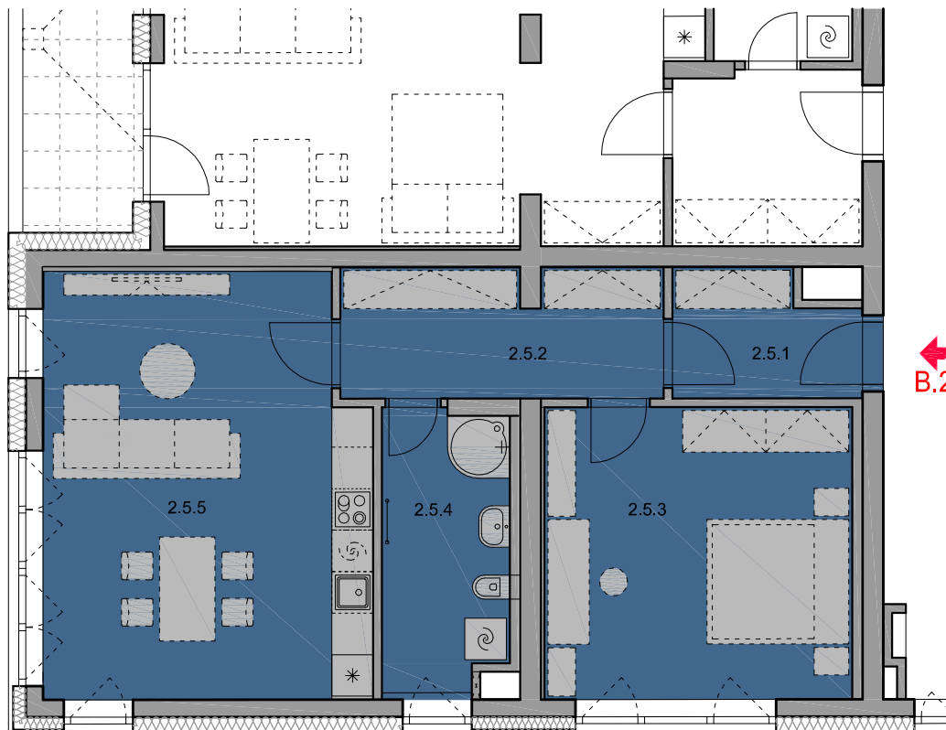
PŮDORYS 1:100
