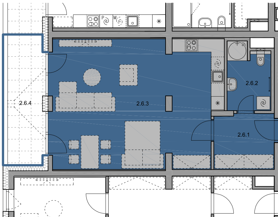
PŮDORYS 1:100
