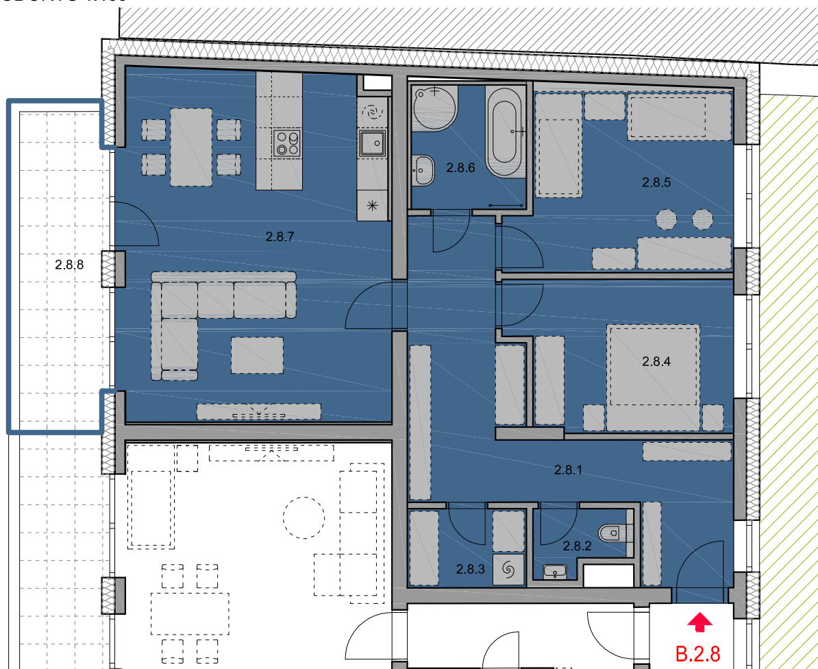
PŮDORYS 1:100
