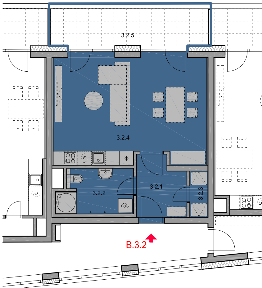
PŮDORYS 1:100
