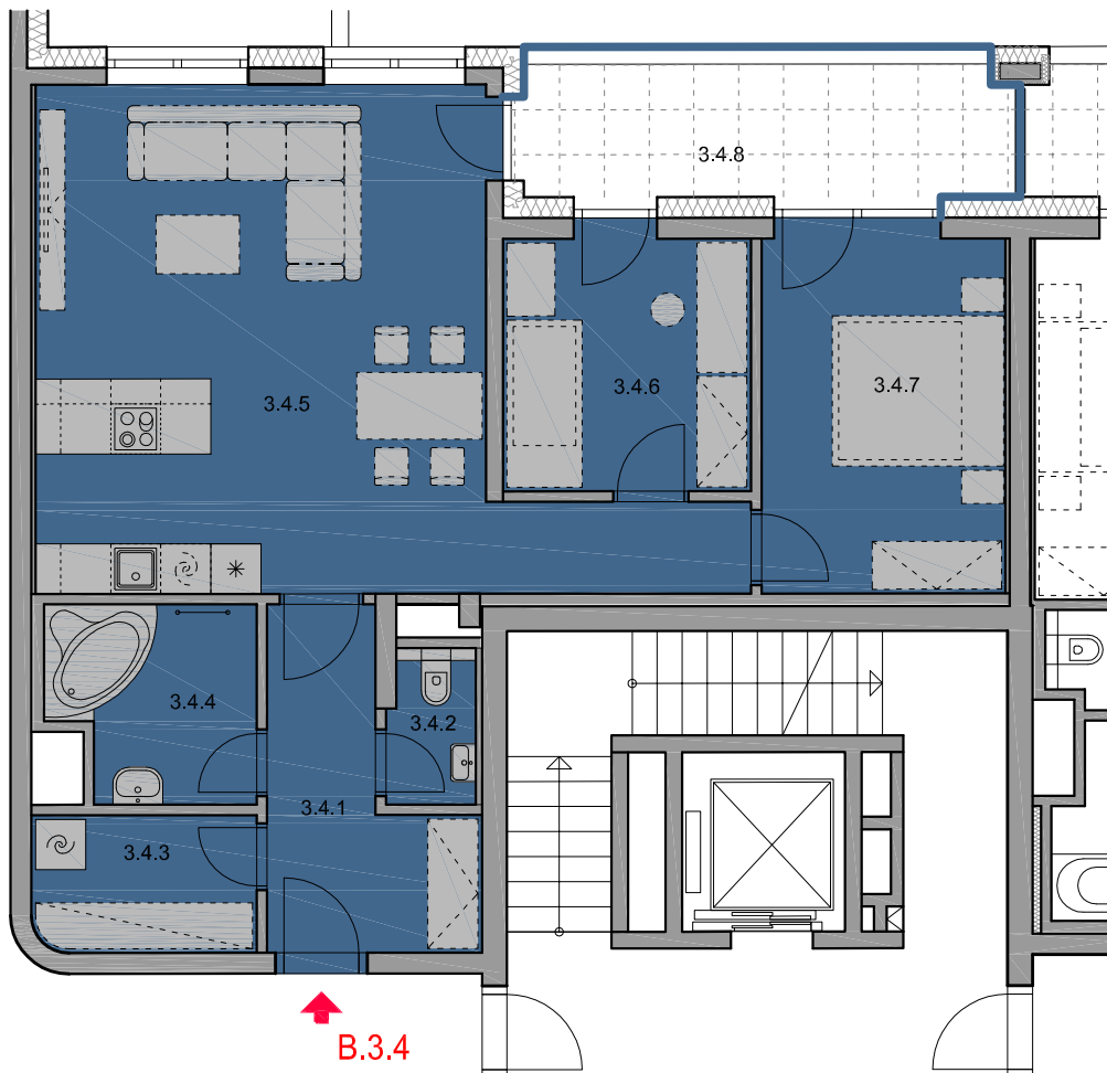
PŮDORYS 1:100
