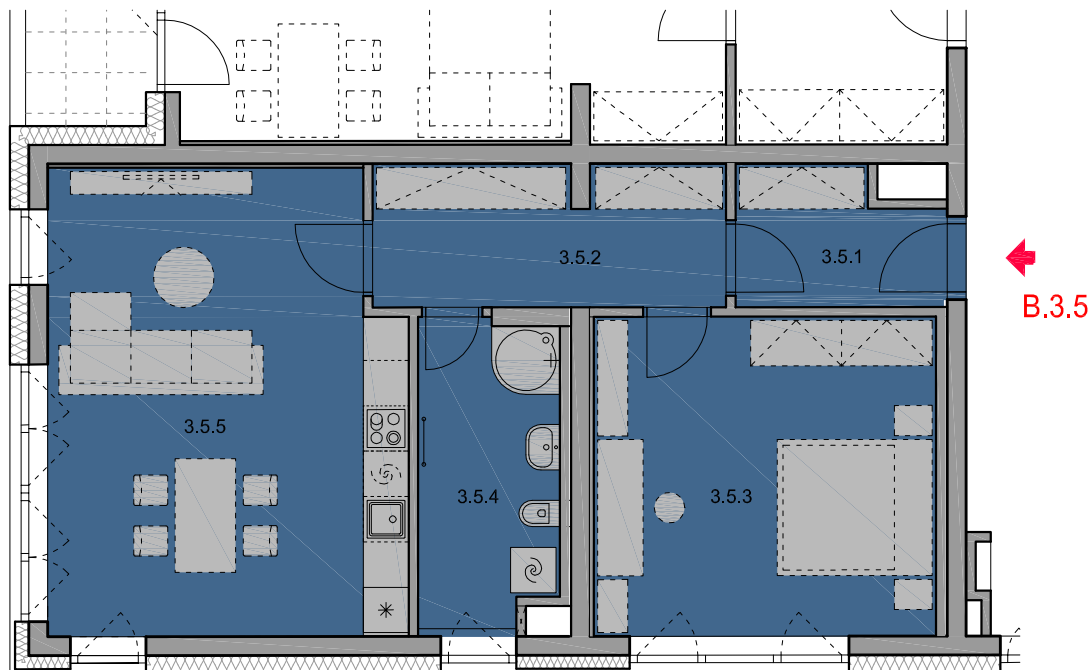
PŮDORYS 1:100
