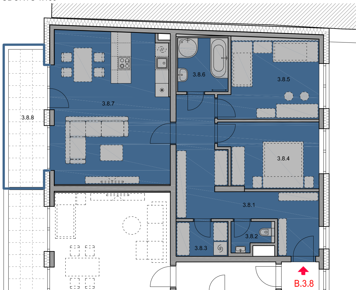
PŮDORYS 1:100
