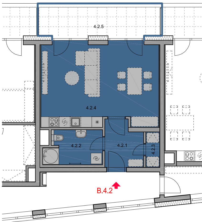
PŮDORYS 1:100
