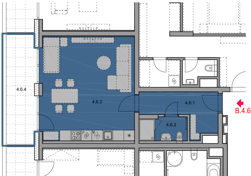
PŮDORYS 1:100
