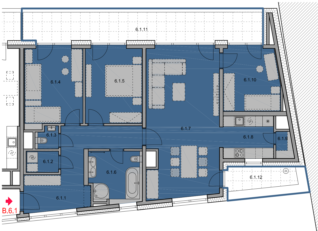
PŮDORYS 1:100
