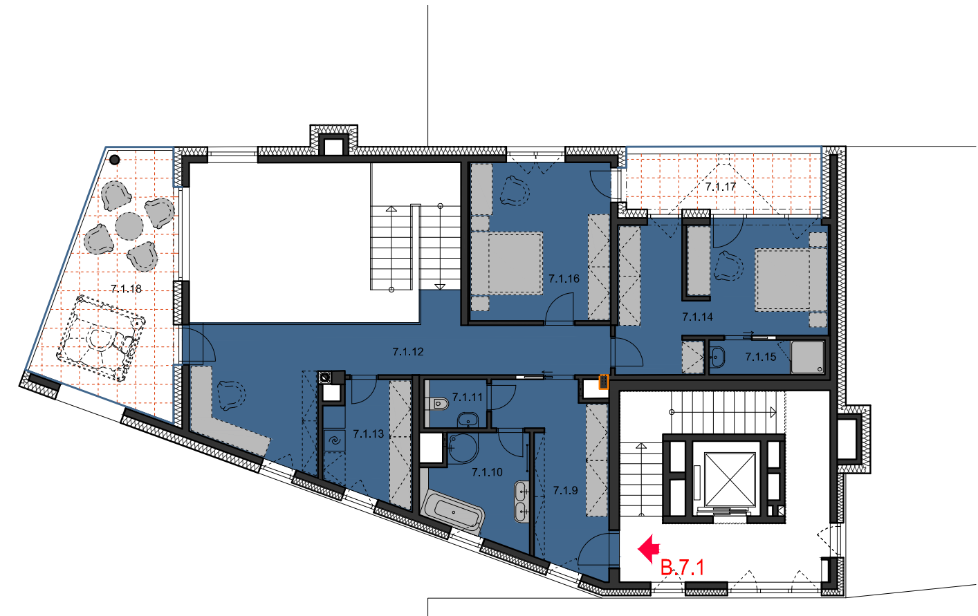
PŮDORYS 8.NP 1:150
