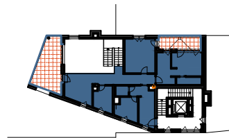
SCHEMATICKÝ PŮDORYS 8.NP
