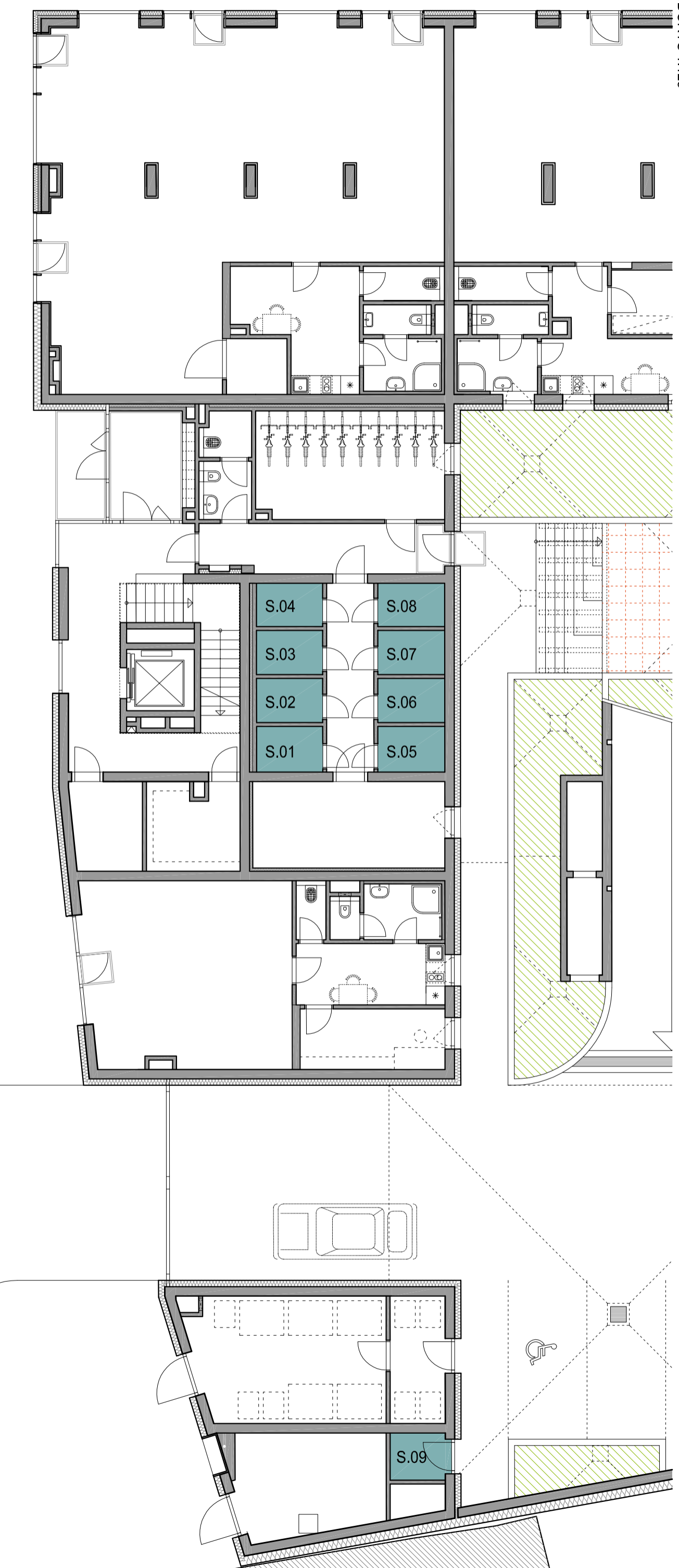
PŮDORYS 1:125
